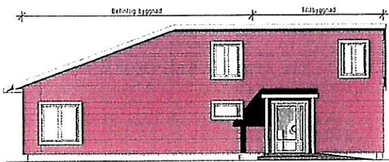
Fasad Öster
