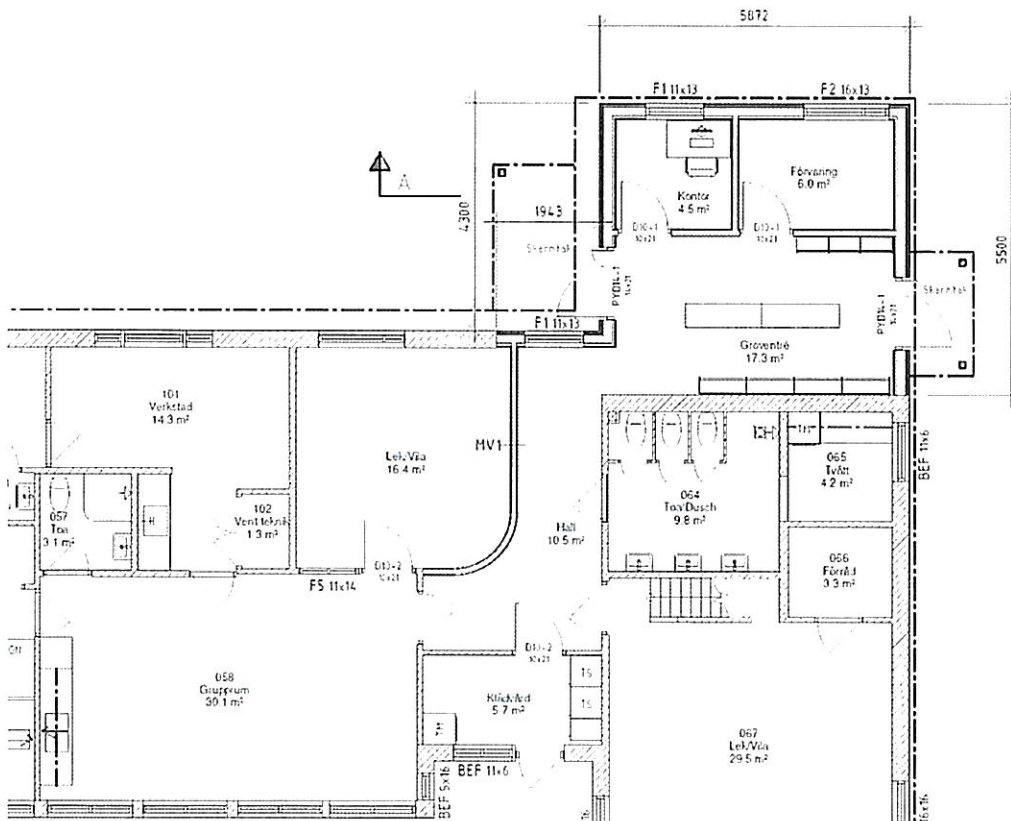
Ritning 2 – planlösning tillbyggnad daghem (Byggkontroll AB, 2023)
